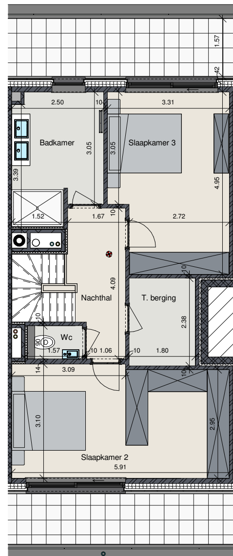
Verdieping 0 1 2 3 4 5 Meter
